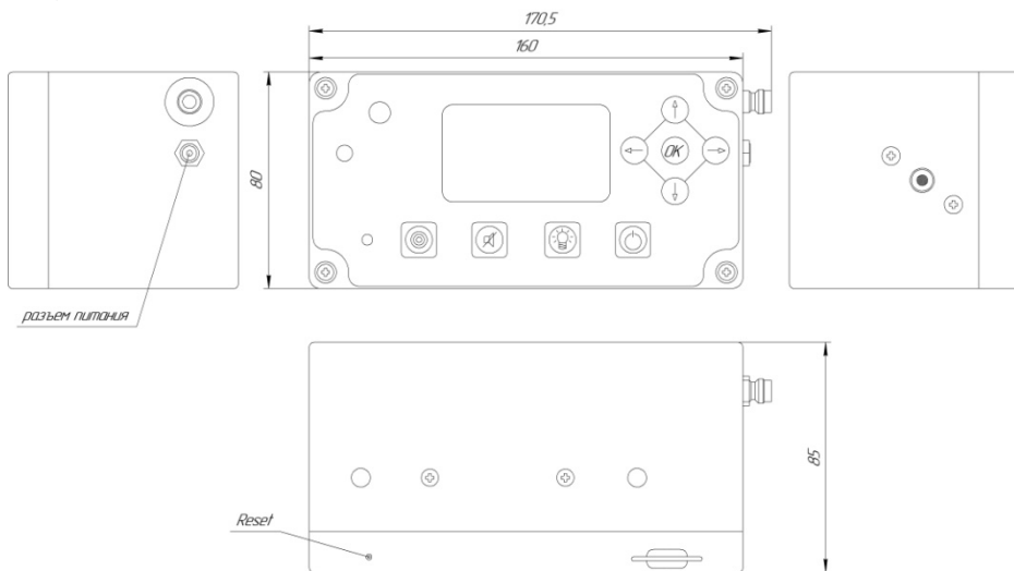
Рисунок 1. Габаритный черт ёж прибора
